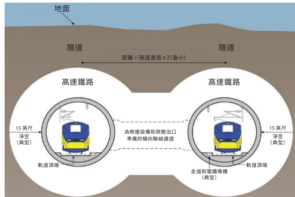
圖 2. 圖解橫截面顯示雙孔隧道的典型配置。
